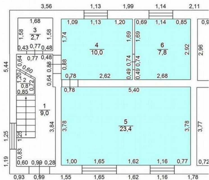
Первый этаж помещения 1 S=41.2 m2
