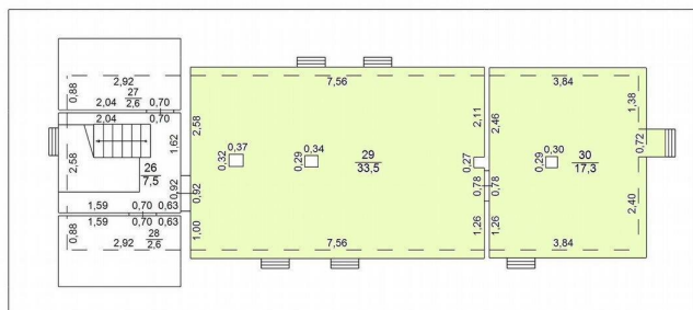
Третий этаж S=50.8 m2
